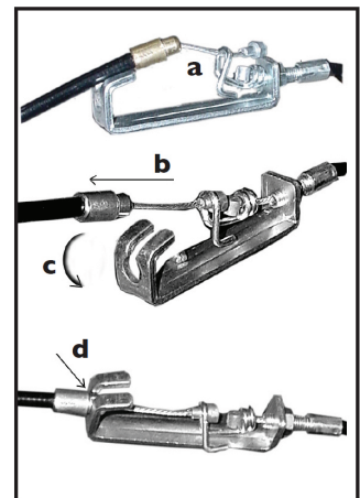
Βήματα σύνδεσης ντιζας
