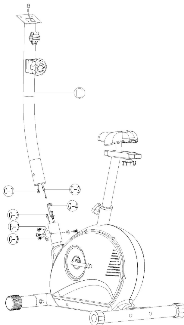
Sequenza di fissaggio del tirante con l'attacco
